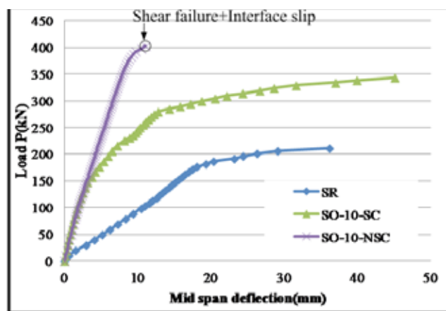
تصویر ۸: رابطه بین بار و انحراف مرکزی سری ۲ آزمایش‌ها. مأخذ: نگارندگان.
