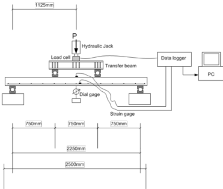
تصویر ۵: طرح آزمایش نمونه تاول. مأخذ: نگارندگان.
