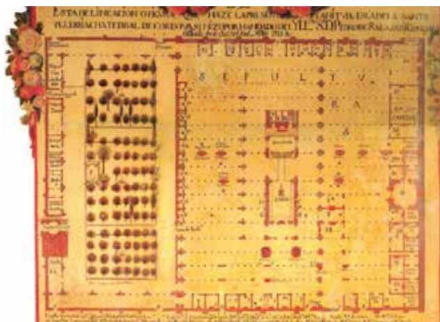
تصویر ۲. پلان کلیسای جامع کوردوبا که در سال ۱۷۴۱ میلادی ترسیم شده است. نارانجستان این کلیسا در تصویر دیده می‌شود. مأخذ: Ruggles, 2008.
