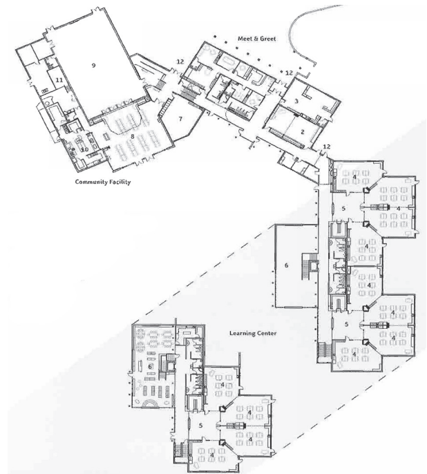
تصویر ۴: پلان مدرسه ابتدایی ایگل راک. مأخذ: Ford, 2007.
