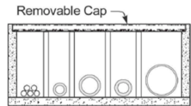
سازه‌های راهرویی تأسیسات شهری در اندازه کوچکتر با مسیر دسترسی محدود
