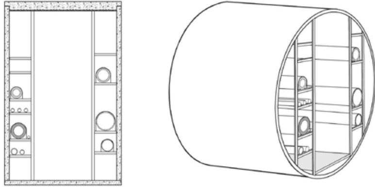
دو نمونه از سازه‌های راهرویی تأسیسات شهری با مسیر دسترسی آندرو
