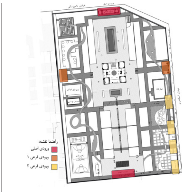
تصویر ۱۸: نقشه ورودی‌های باغ ایرانی دامیرشکی. مأخذ: مهندسین مشاور پژوهشکده نظر.
